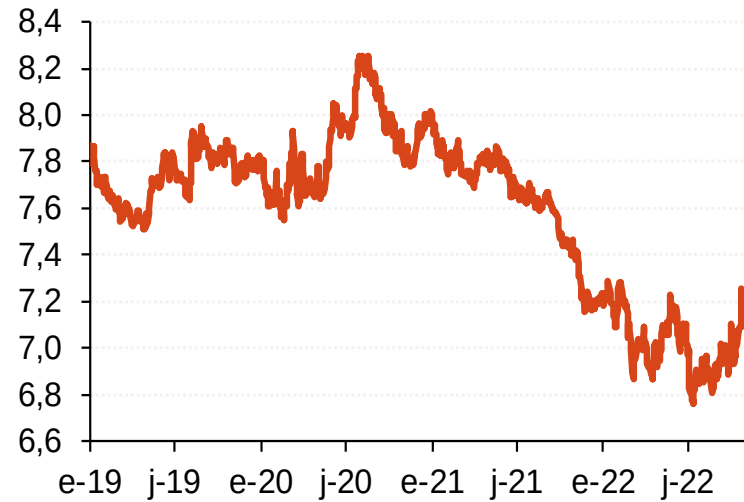
CNY/EUR
