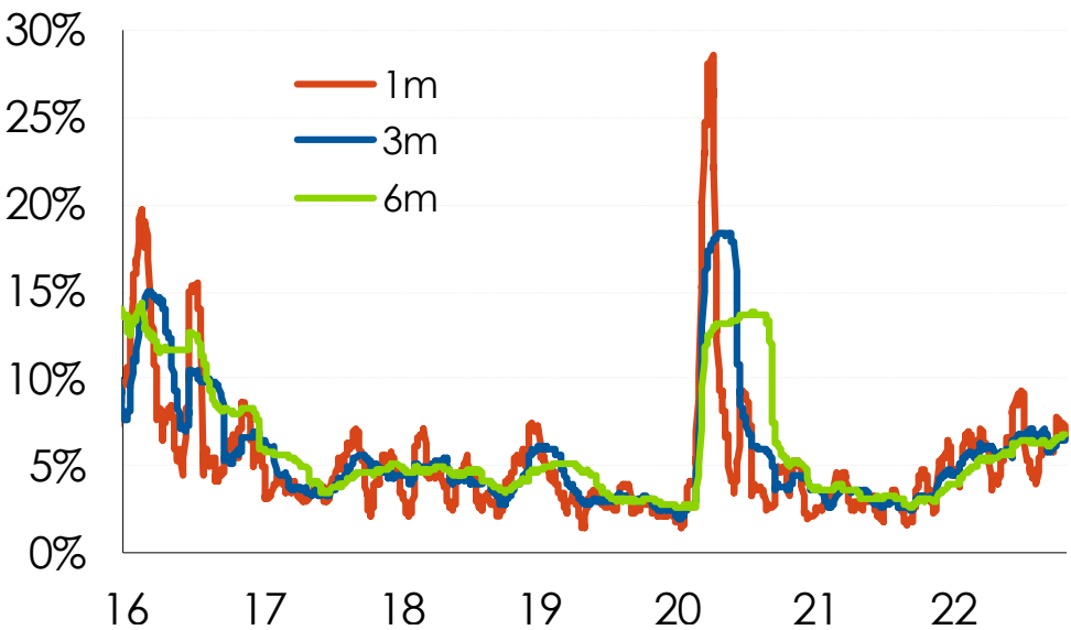
Volatilidad
