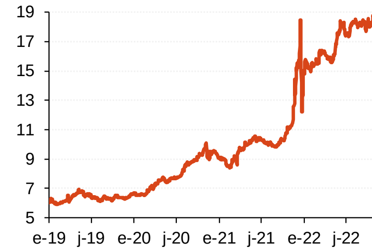
TRY/EUR
