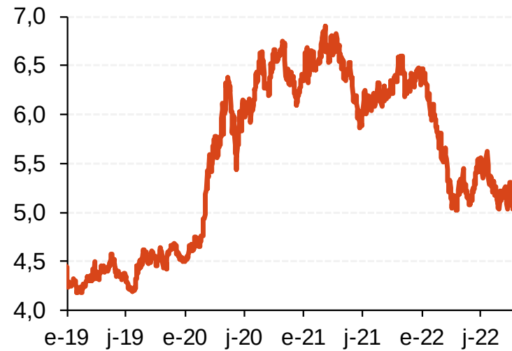
BRL/EUR
