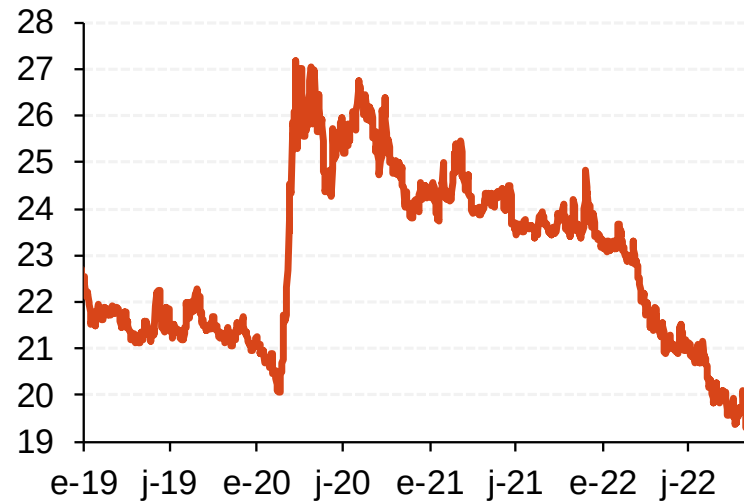
MXN/EUR
