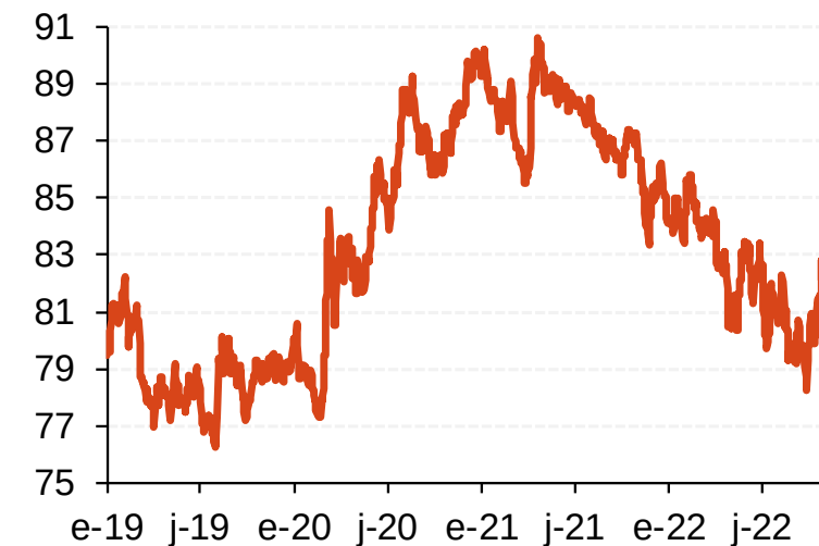
INR/EUR
